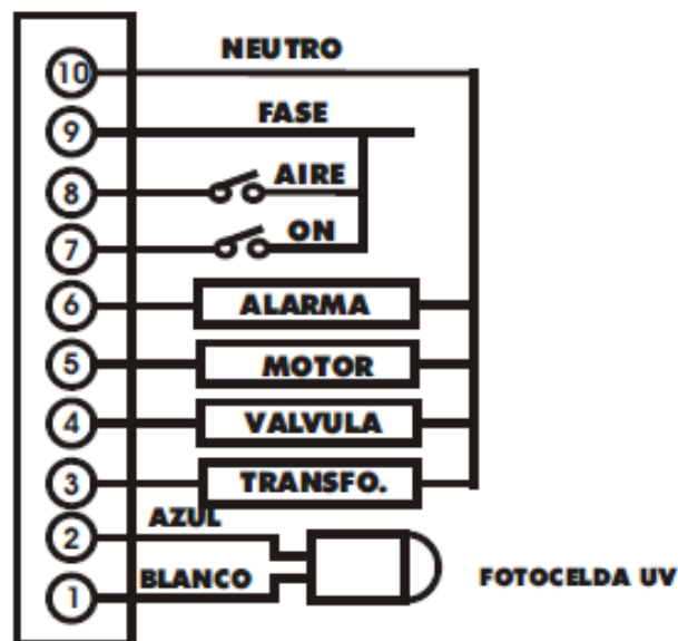
Fig 3 Diagrama de conexión PQ 3003
