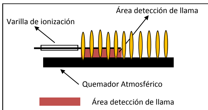
Fig 6 Forma de colocación varilla de ionización PA 4001
