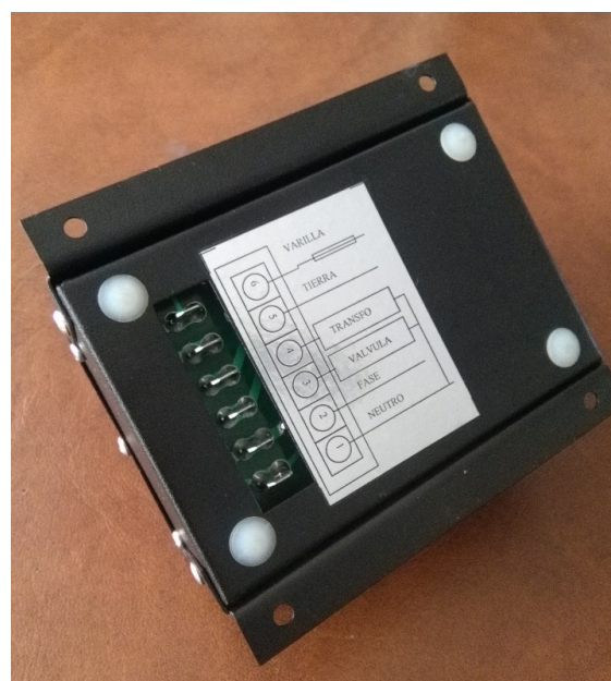
Fig 3 Foto frontal PA 4001
