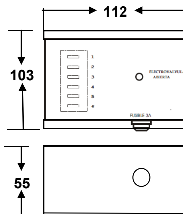
Fig 9 Dimensiones PA 4001
