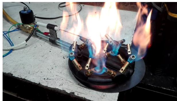
Fig 8 Foto colocación varilla de ionización PA 4001
