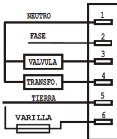
Fig 4 Diagrama de conexión PA 4001
